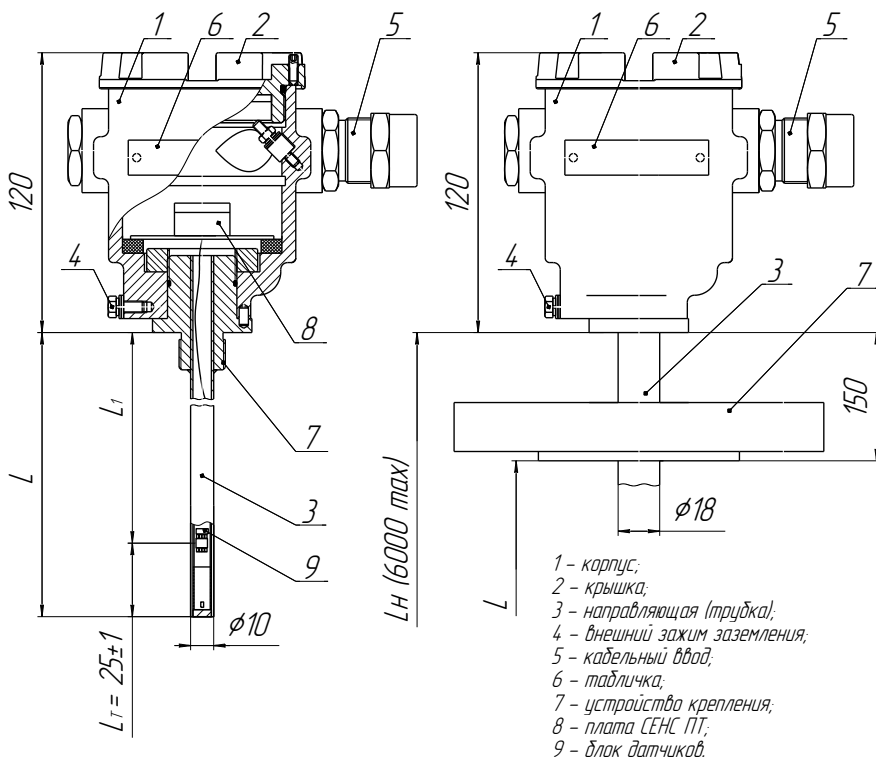
Рисунок 1 – СЕНС ПТ и СЕНС ПТ-Modbus
